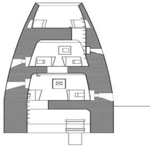
說明：外埔村砲台牆體與樓板剖面
